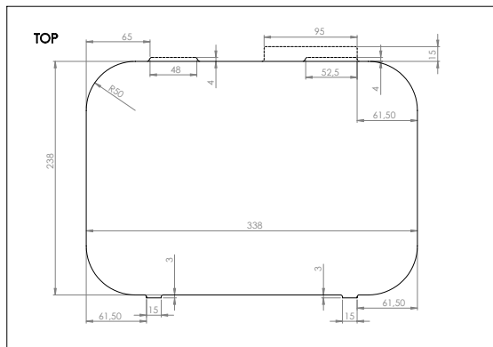
Draufsicht Arbeitsplatte
