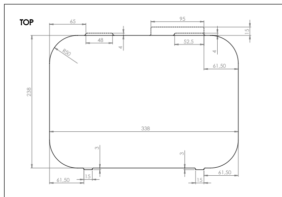
Bovenaanzicht werkblad
