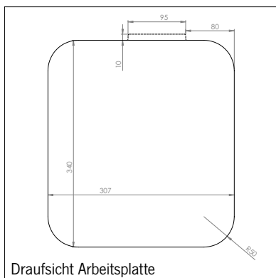
Draufsicht Arbeitsplatte
